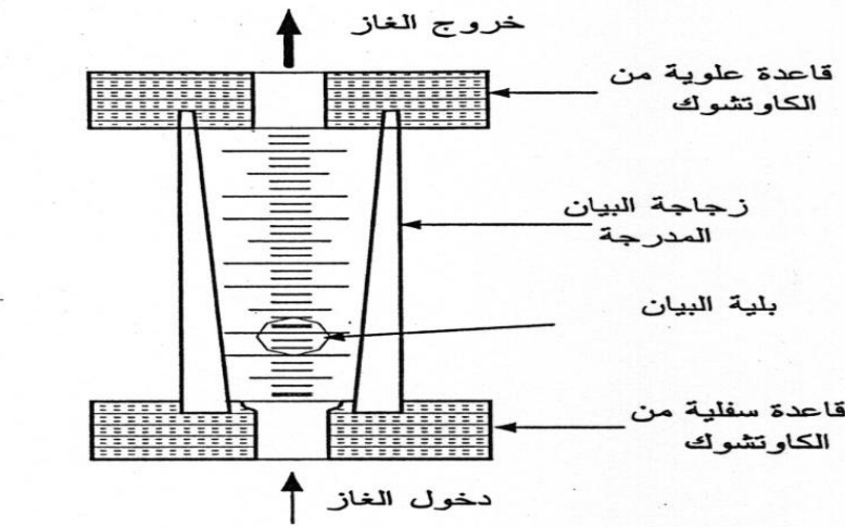
شكل ( ٢-٩ ) مقياس التدفق
