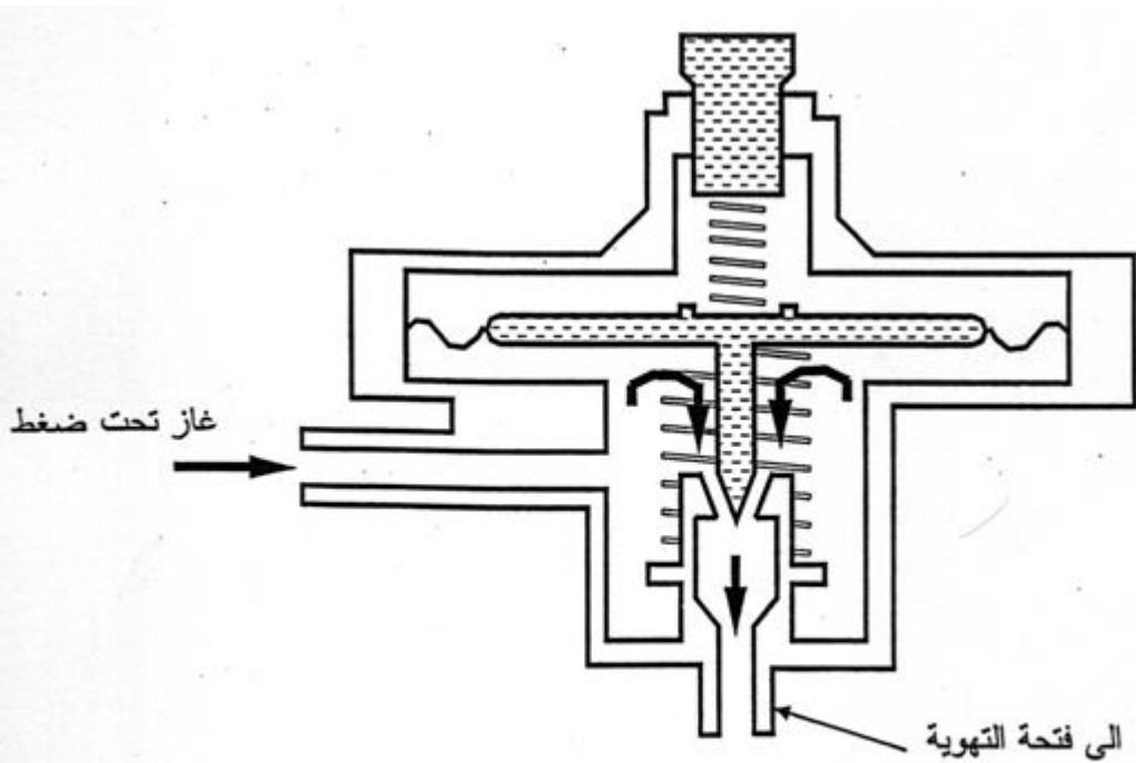
شكل رقم (٢-١٣) (36) كيفية عمل صمام تحرير الضغط
