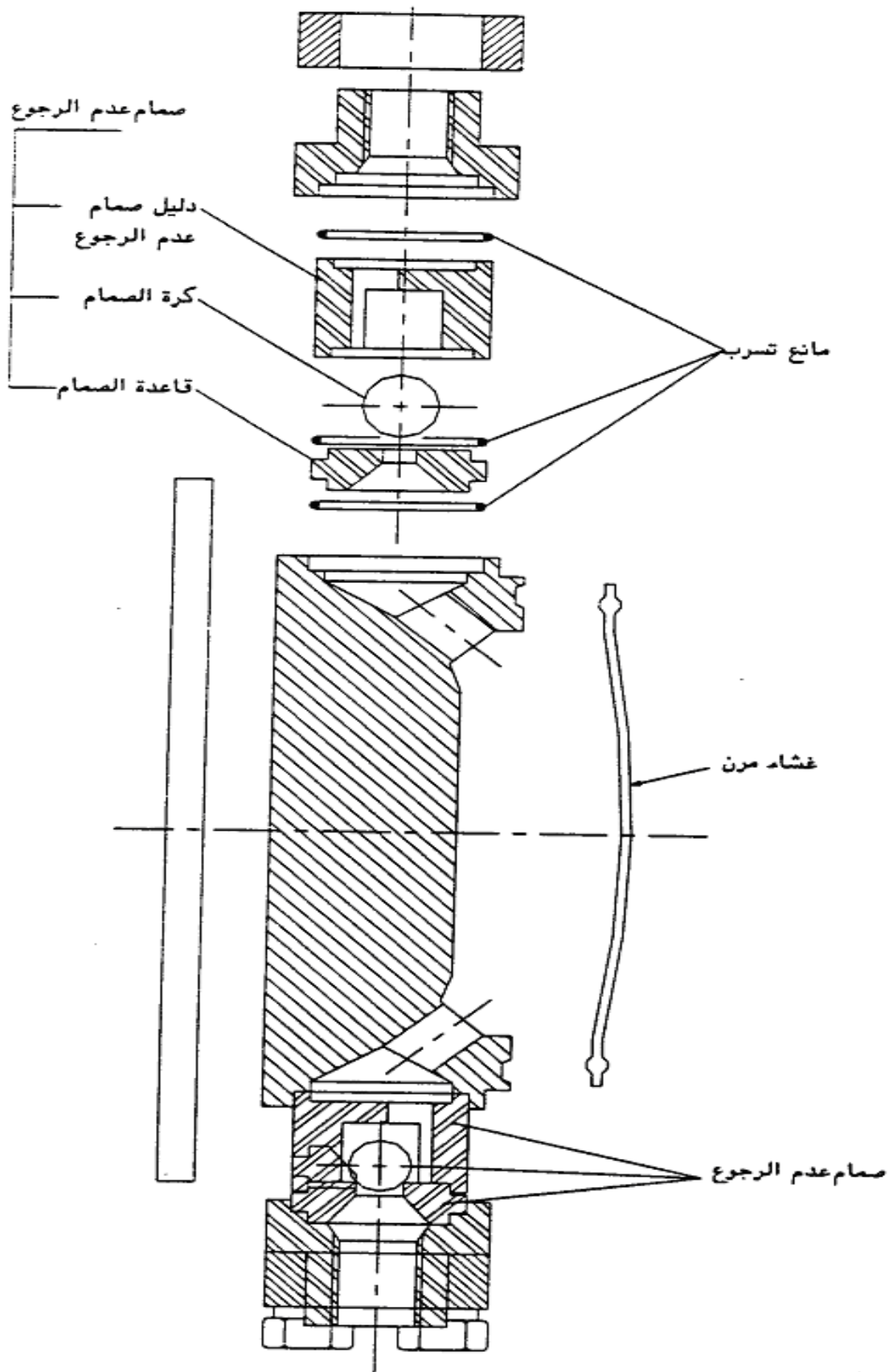
شكل رقم (5-8) تفاصيل الظلمبة ذات الغشاء
