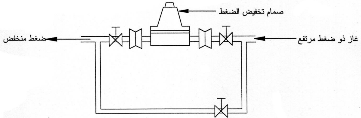
شكل رقم (٣-٢) 21 صمام تخفيض الضغط وإيقاف الكلور
