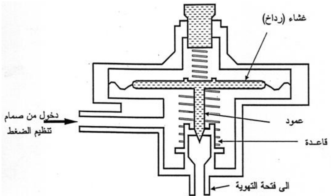
شكل رقم (٢-١٢) (35) صمام تحرير الضغط
