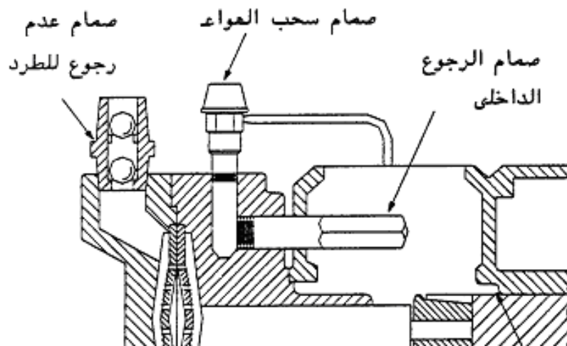
الشكل رقم (1) طلمبة اضافة محلول كبريتات الالومنيوم (الشبة) ذات المكبس رجوع للسحب
