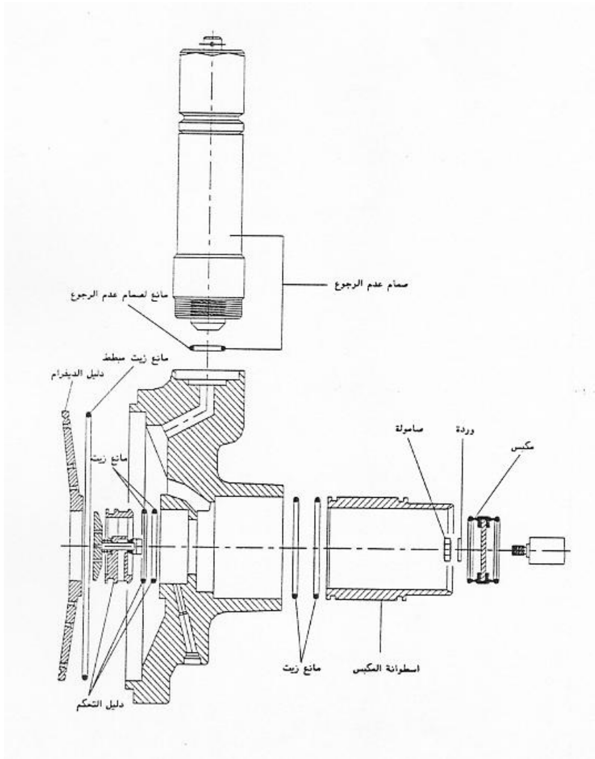
شكل رقم ( 9 ) التفاصيل الميكانيكية لطلمبة ذات الغشاء (الرق)
