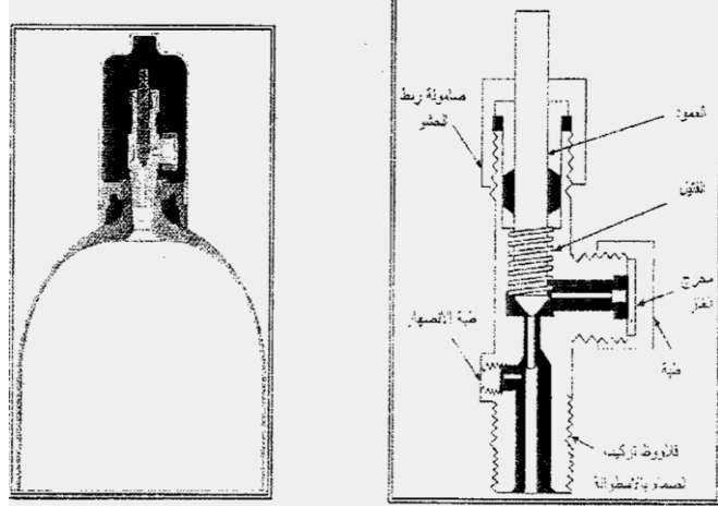
شكل رقم (٣) صمام (محبس) أسطوانة كلور سعة ٥٠ كجم
