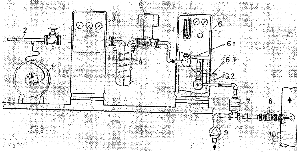
شكل رقم (١٩) شكل يوضح ترتيب جهاز الكلور ضمن النظام
