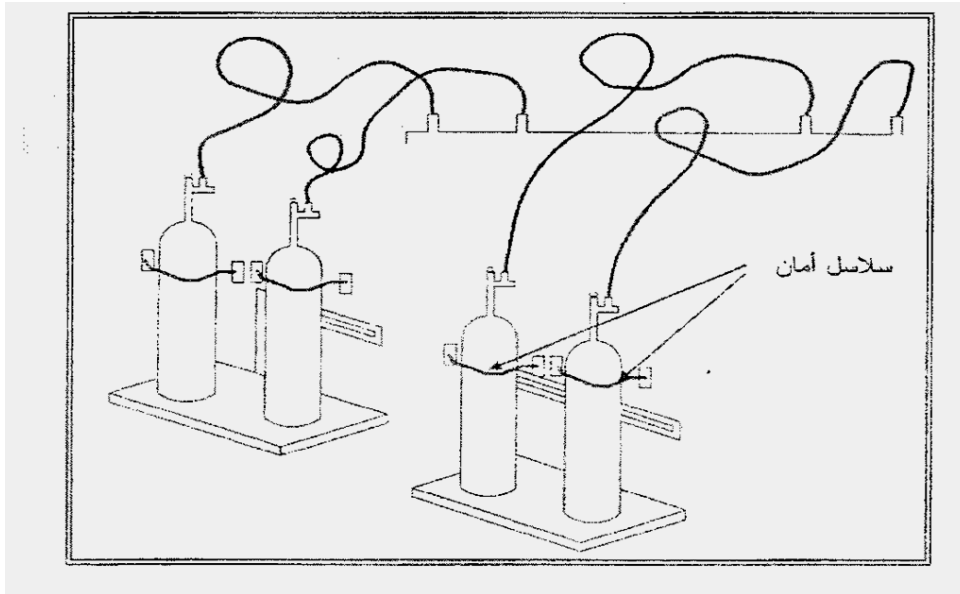
شكل رقم (٥) تثبيت الأسطوانات بالسلاسل حماية لها من السقوط
