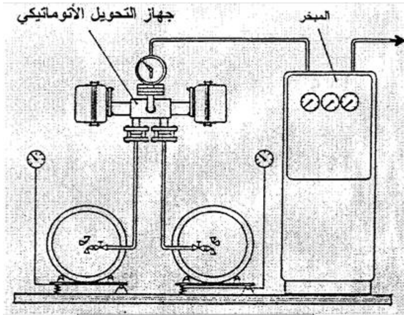
شكل رقم (10) وضع جهاز التحويل في النظام
