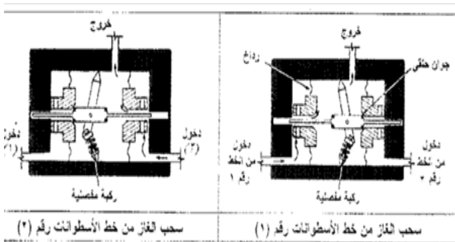
شكل رقم (11) نموذج يوضح مكونات جهاز التحويل وطريقة عمله
