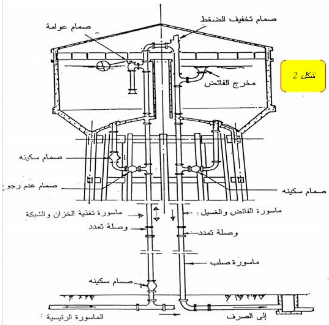
شكل رقم (28) توصيلات الخزان العالي
