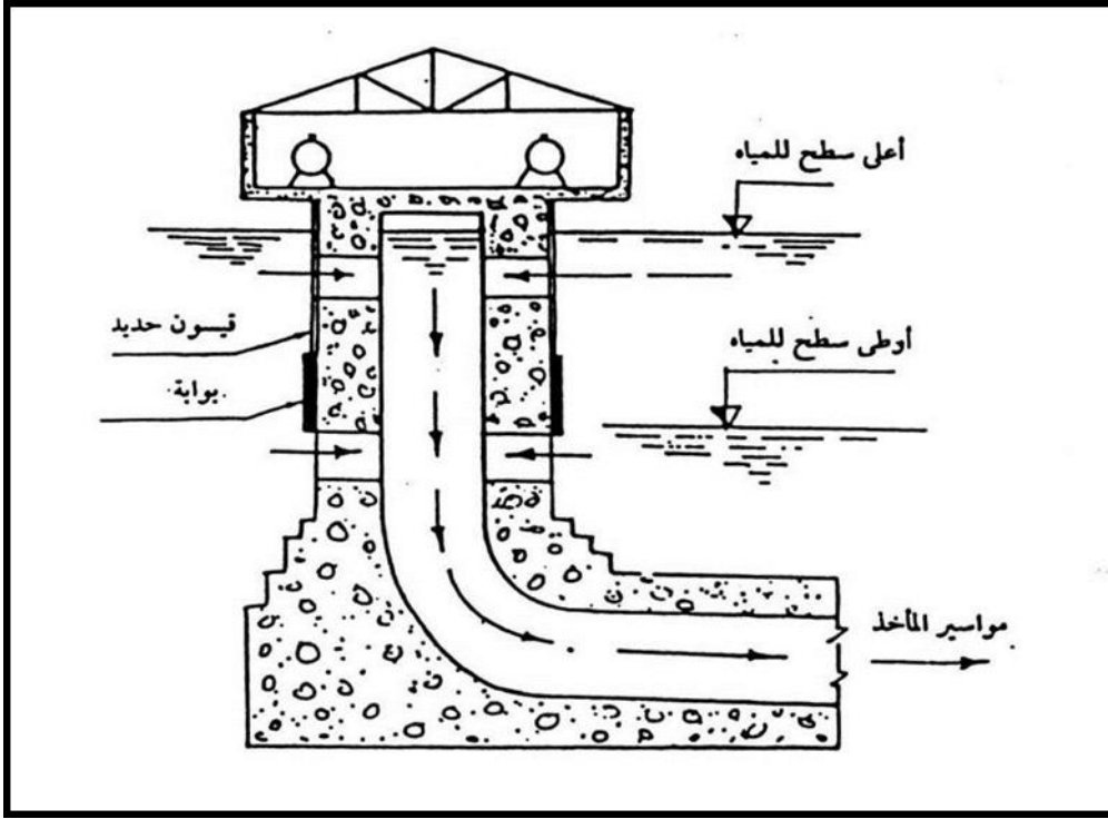
شكل رقم ( 4 ) مأخذ برج
