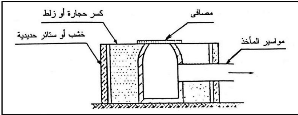
شكل رقم ( 3 ) مأخذ عميق
