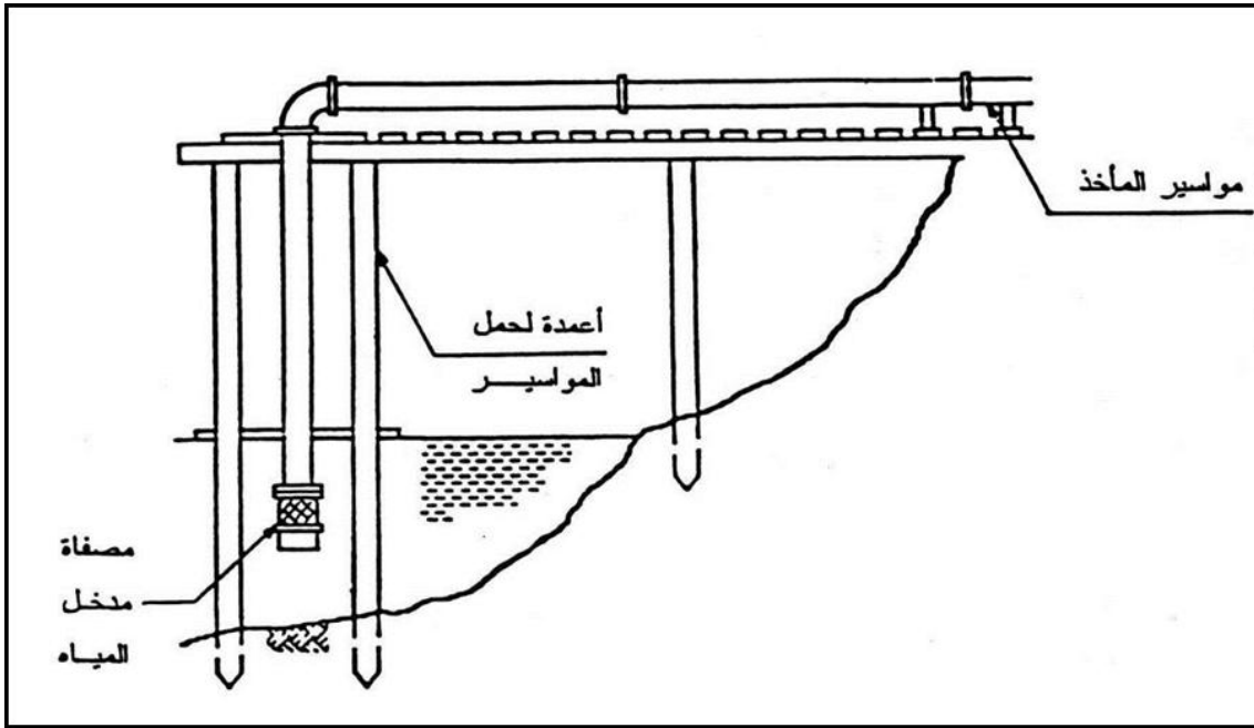
شكل رقم (1) مآخذ ماسورة يستخدم في أعمال التنقية
