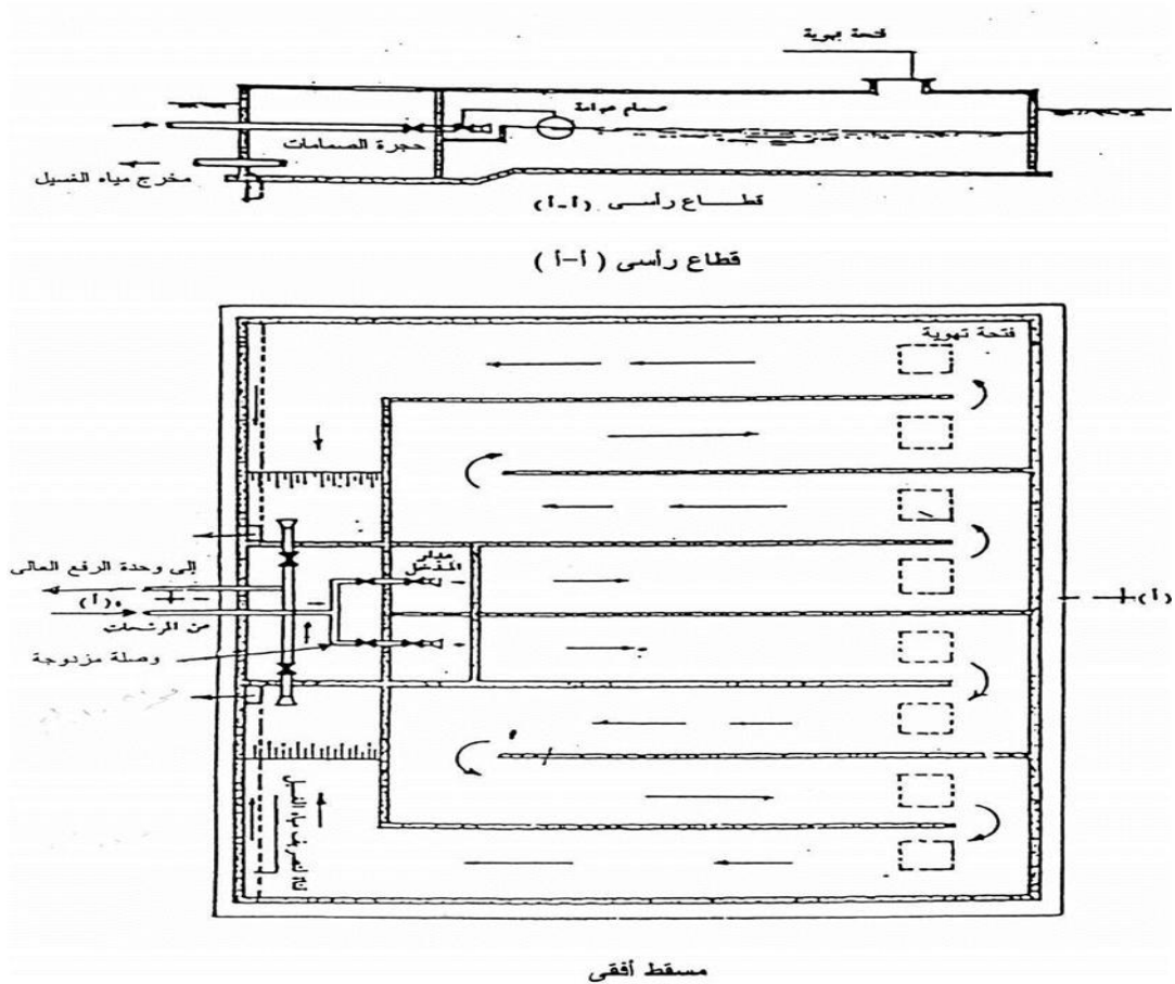
شكل رقم ( 27 ) مسقط افقى للخزان لأرضى
