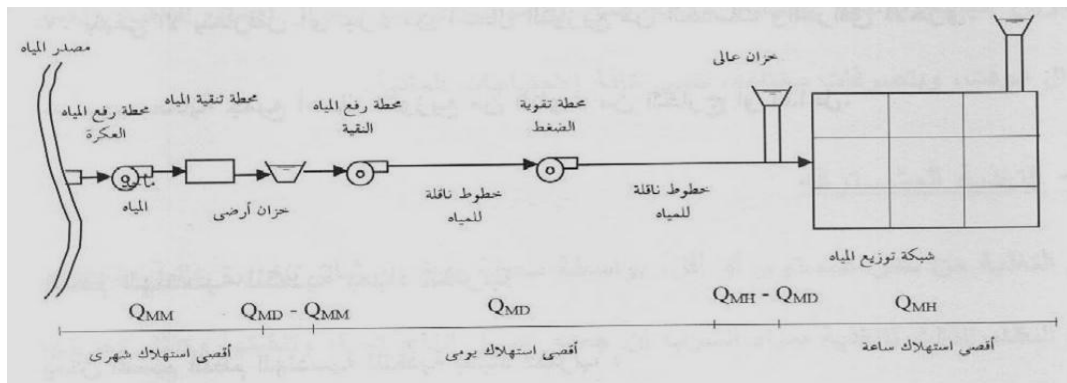
شكل رقم ( 29 ) تخطيط شبكات توزيع مياه الشرب
