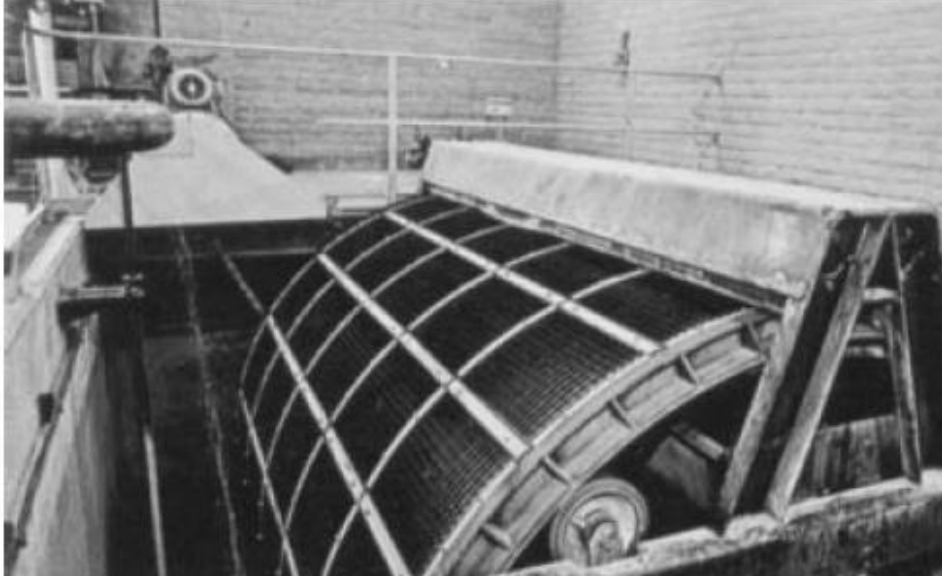
شكل رقم (6) المصافي الدقيقة
