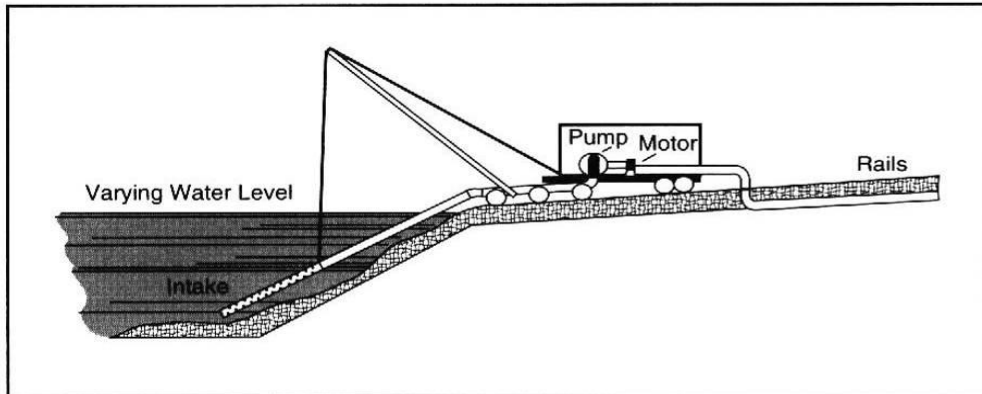
شكل رقم ( 5 ) مأخذ مؤقت
