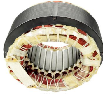
العضو الثابت
