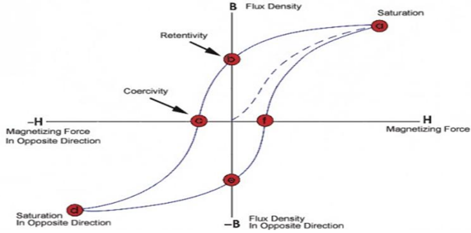
شكل رقم (4) يوضح منحنى التخلف المغناطيسي
