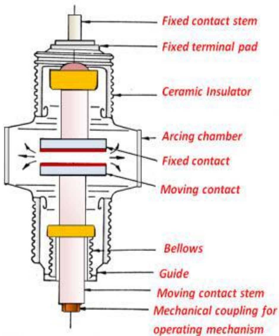
شكل "4" قاطع مفرغ من الهواء " طراز اجيماك "
