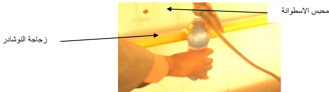
الصورة توضح طريقة الكشف عن مكان تسريب الكلور باستخدام النشادر
