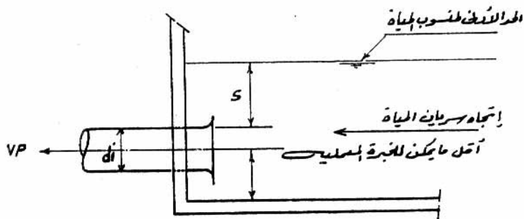
شكل (٢-٢٨) أقل عمق للمياه بالبيارة
