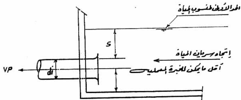
شكل (٢٨-٢) أقل عمق للمياه بالبيارة
