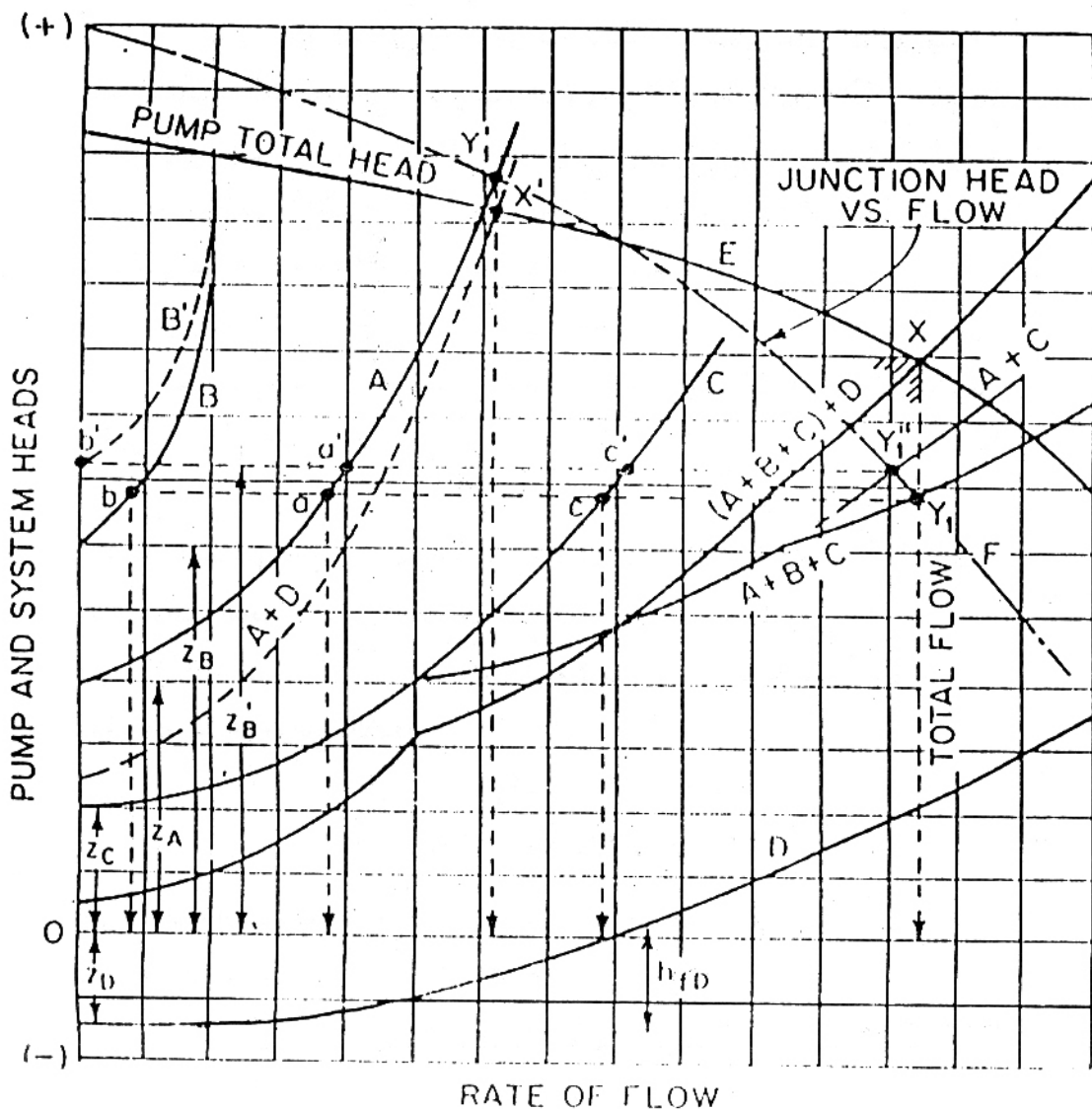
شكل (٨-٢) منحنى أداء المنظومة الموضحة فى شكل (٧-٢)
