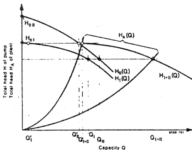
شكل (٢-١٣) منحنى اداء طلمبتين مختلفتين فى الرفع منفردتين ومجتمعين على التوازي
