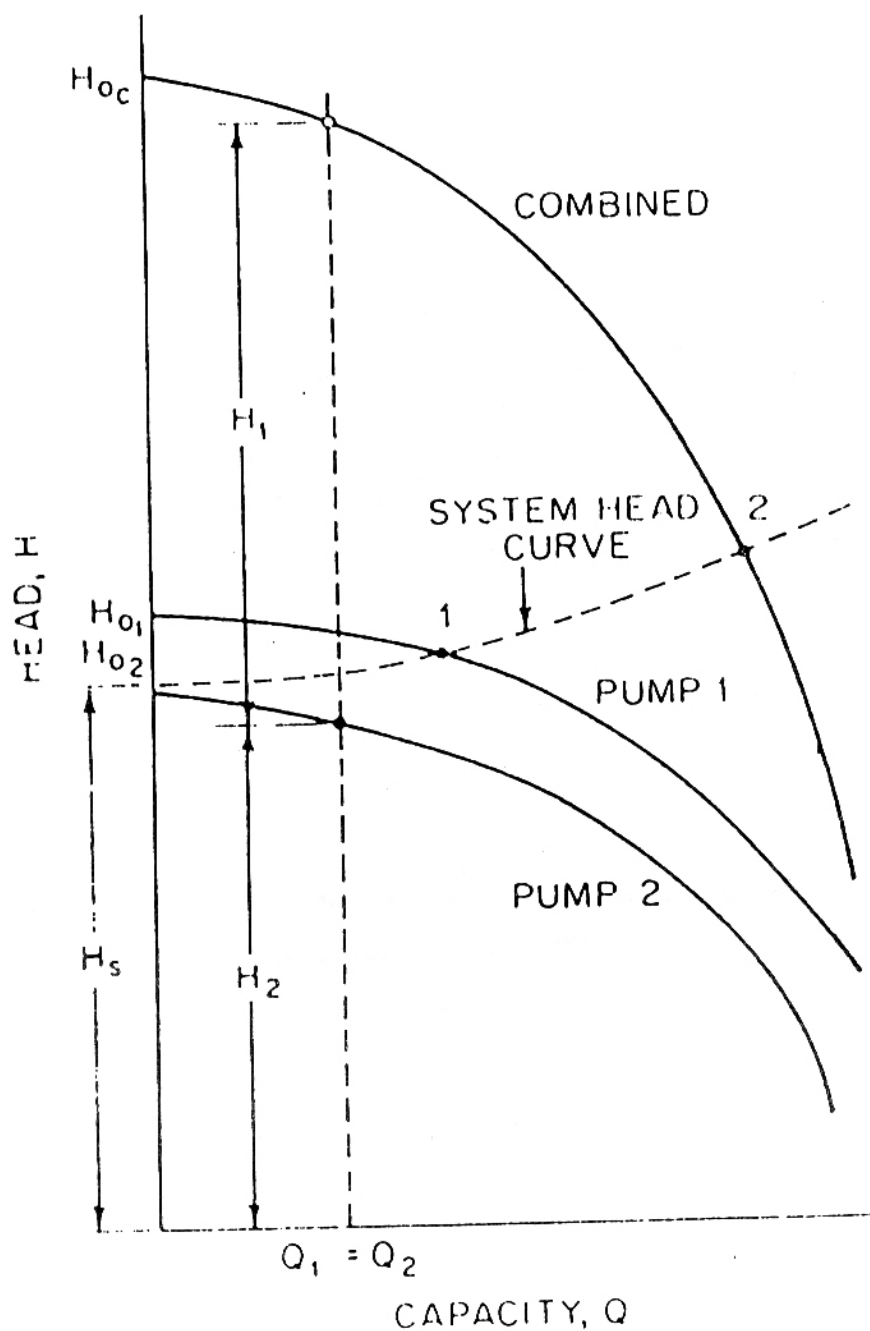
شكل (٢-١٦) منحنيات أداء ظلميتين منفردتين ومجتمعتين على التوالي
