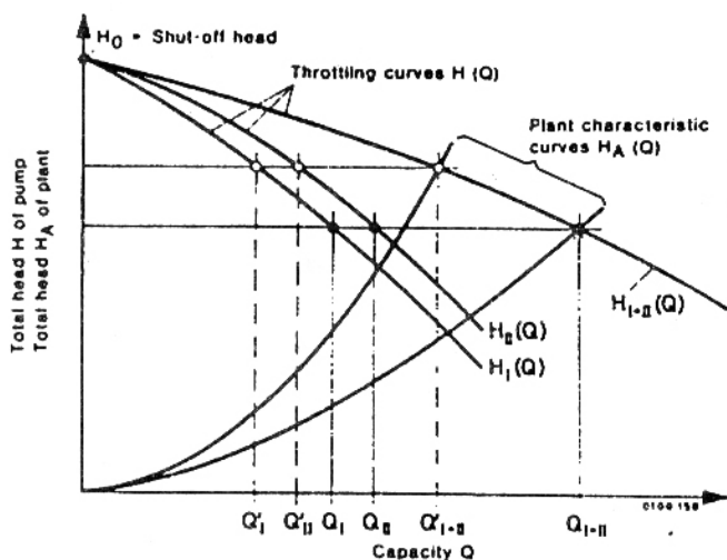
شكل (١٢-٢) منحنى تشغيل ظلمبتين على التوالى مجتمعين
