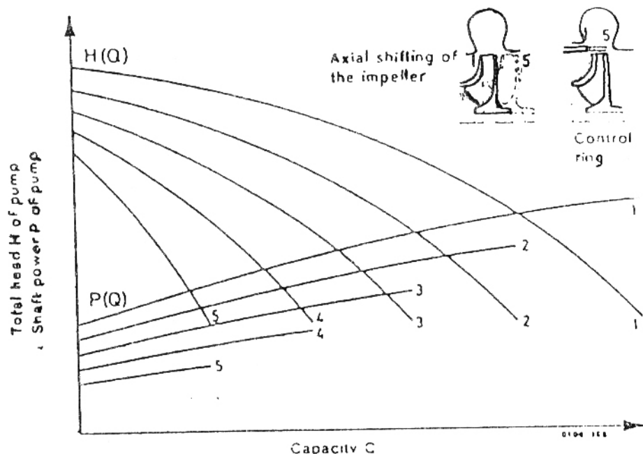
شكل (٢-٢٠) تغيير منحنيات الخواص نتيجة تغيير وضع المروحة أو إضافة غطاء حاكم فى مدخل الغلاف الحلزوني
