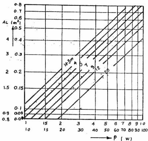
شكل (٣-٣) نموذج ارام تحديد مساحة فتحتى دخول وخروج الهواء
