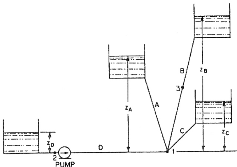
شكل (٧-٢) نظام مكون من خزان سحب وخط مواسير رئيسي وخطوط فرعية مختلفة وكل منها ينتهي بخزان إستقبال
