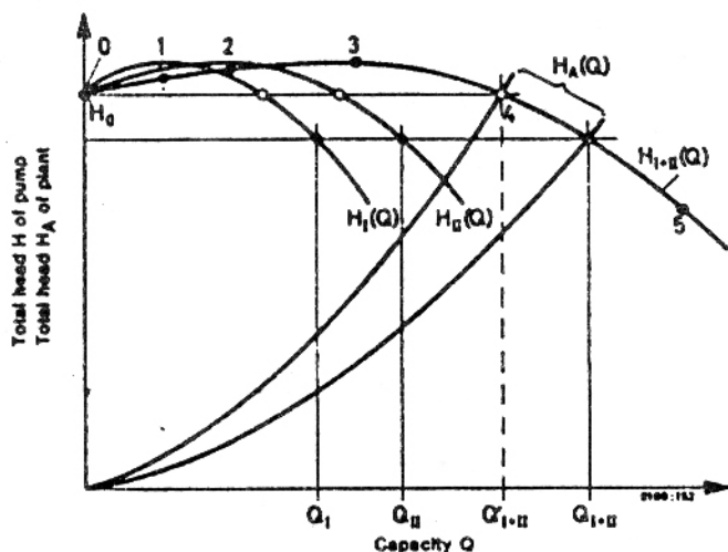
شكل (٢-١٤) منحنيات غير مستقرة لطلمبتين مختلفتين الخواص والرفع الاقصى واحد لكل منهما ومجتمعين على التوازي
