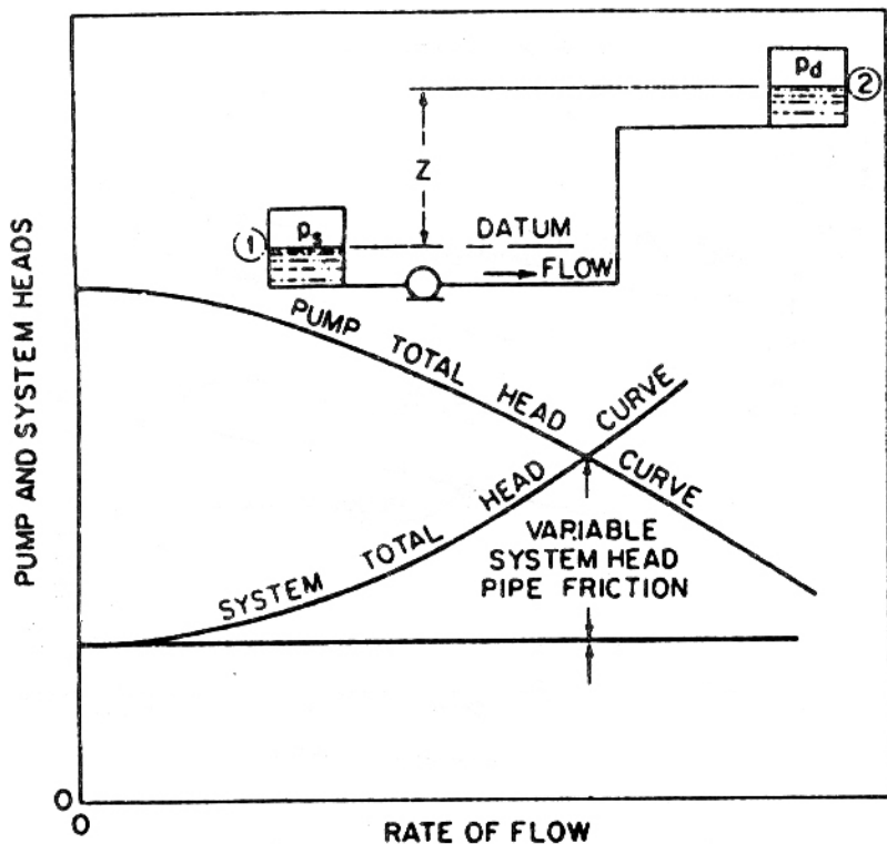
شكل (٢-١) منحنى أداء النظام المكون من خزان سحب وخزان استقبال ومضخة، خط مواسير بينهم
