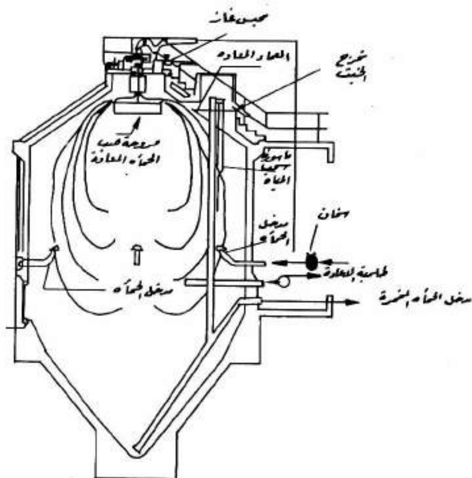
تکلیف (۲-۱۶): مکتوبات منبر الحماة ذو المعدل العالمی
