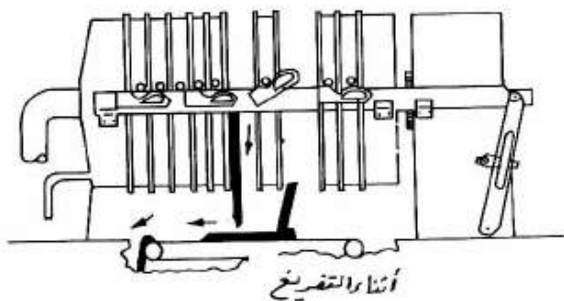
شكل (٢-٢٢): مرشح ماء يعمل بالضغط (Filter Press)
