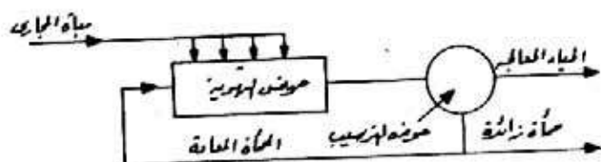
نظام الحمأة المنشطة التقليدية
