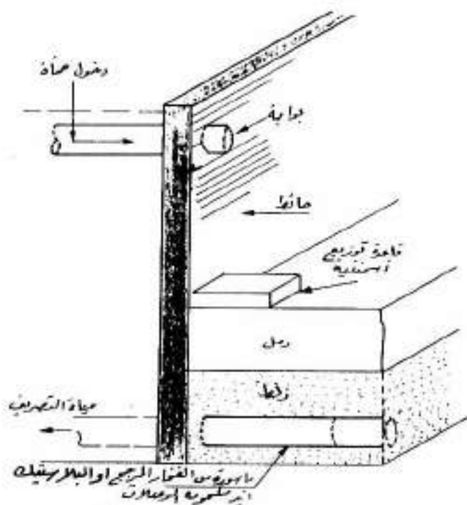
٢- جسم خوض تجفيف المياه
