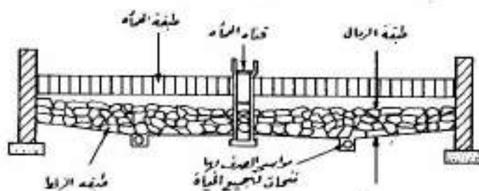
قطاع في أحواض تجفيف المياه
