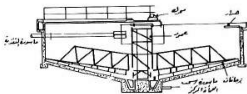
قطاع رأسي ٢-٢
