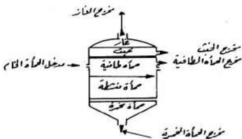
شكل (٢-١٥): مخرج الماء الثقيلة التقليدي
