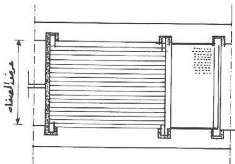
شكل رقم (١-٢): المصافي اليدوية
