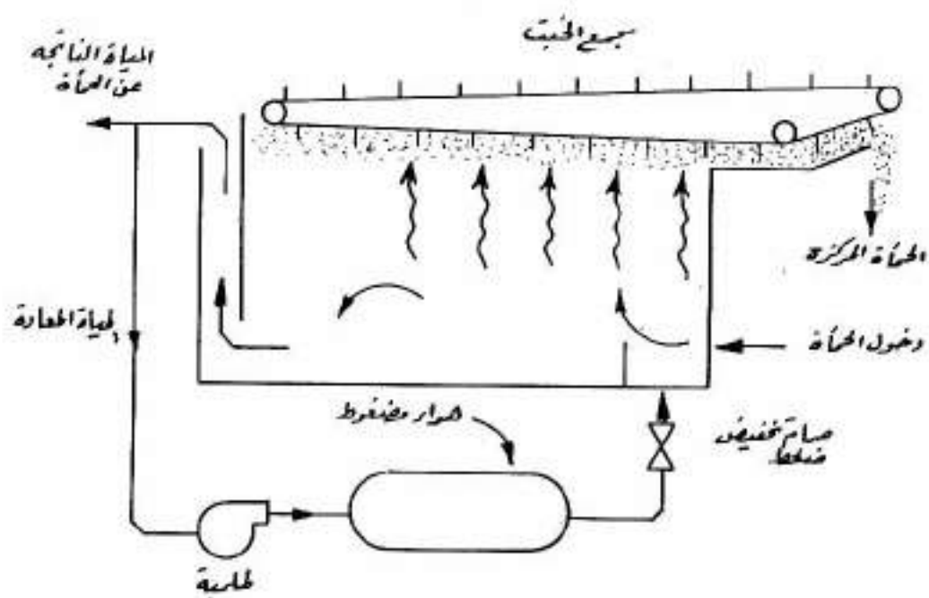
شكل رقم (٢-١٤) تركيز الحساء بالطنوب بواسطة دفع الهواء
