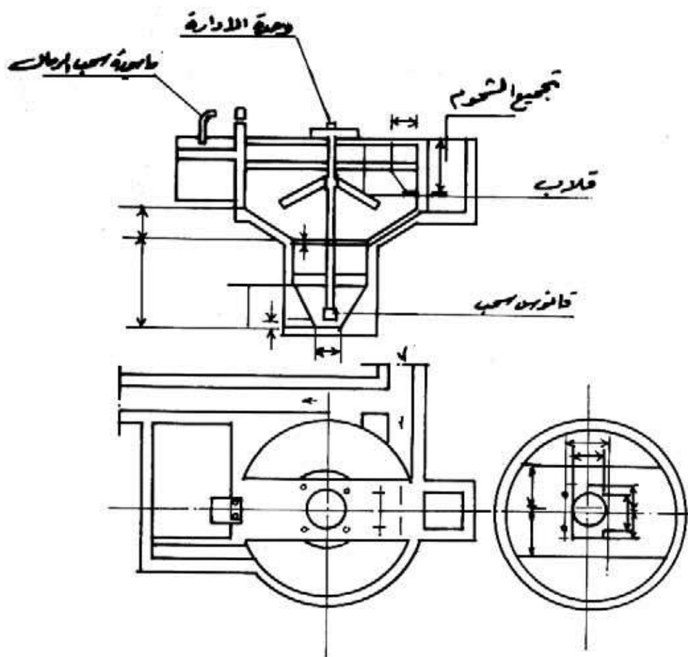
شكل رقم (٢-٢) : حوض فصل الرمال الدائري
