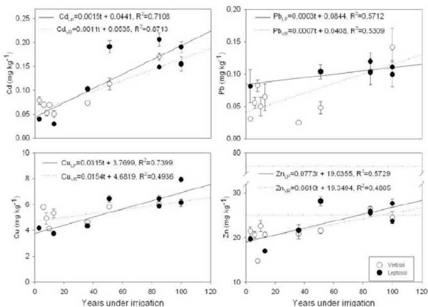
الشكل 4: تراكيز المعادن الثقيلة في البرسيم في الحقول المروية بمياه الصرف الصحي لفترات مختلفة من الزمن (Cayetano-Salazar 2012). VR: Leptosol. LP: Vertisol. البيانات من حقول منطقة Leptosol.
