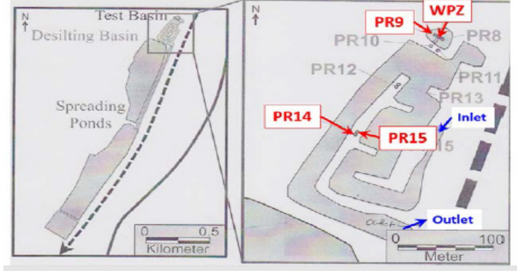
الشكل 3: إعادة تغذية مرفق اختبار حوض يقع في الطرف الشمالي من نهر سان غابرييل للأحواض San Gabriel الساحلية المنتشرة في مونتبييلو فورباي، كاليفورنيا Montebello Forebay, CA (Drewes et al. 2015).
