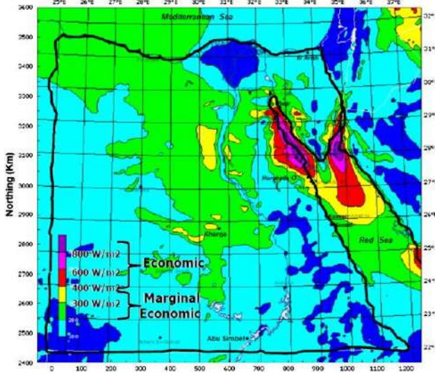
شكل (٦) أطلس الرياح في مصر (كثافة الطاقة عند ٥٠ مترًا، بالوات/م ٢ )
